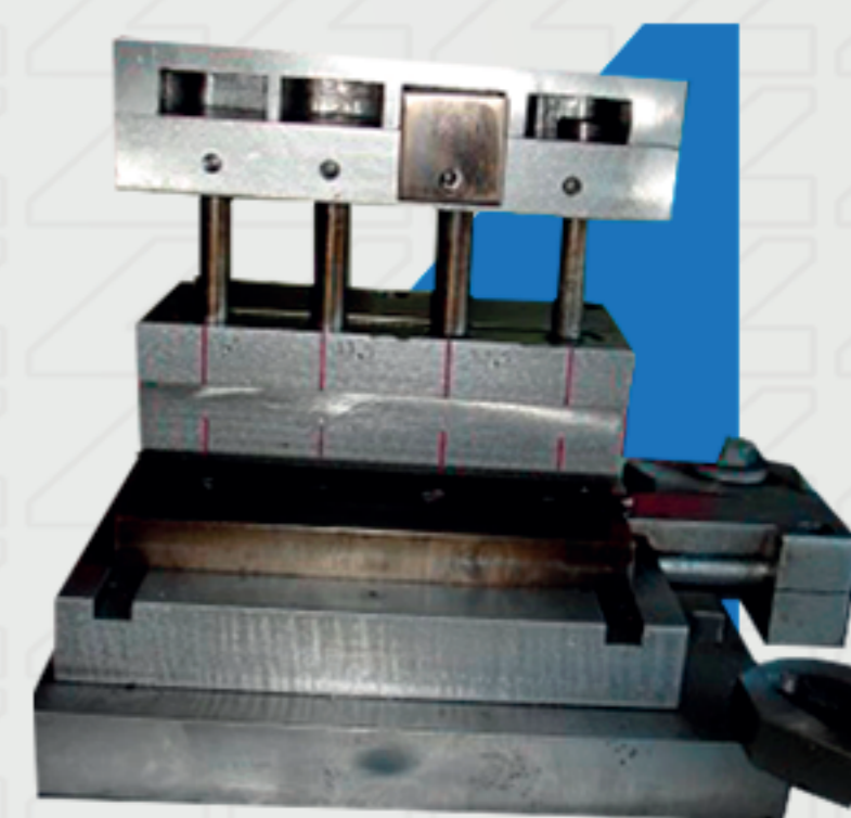
MATRIZ DE FUROS COM SISTEMA NEUTRALIZADOR
