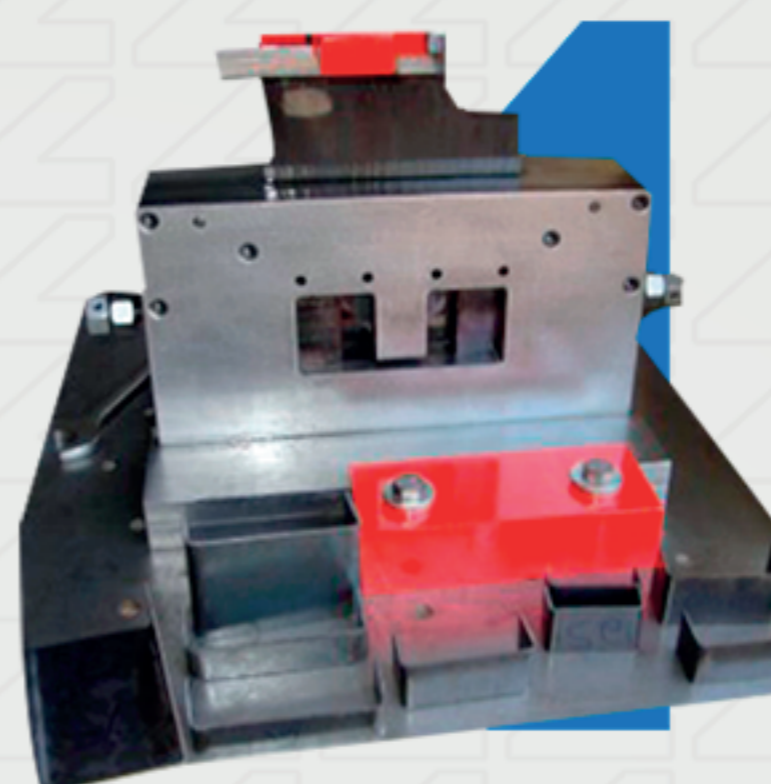
MATRIZ PARA CORTE PERFIL "U"
