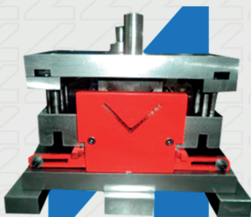
MATRIZ DE CORTE DE CANTONEIRA E FUROS VÁRIAS MEDIDAS
