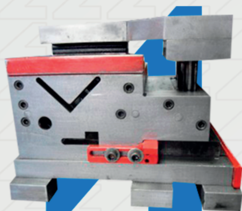
MATRIZ DE CORTE E FUROS
